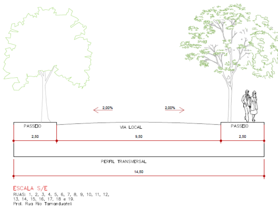
Figura 4. Corte Transversal das Ruas de 14,50 metros.
