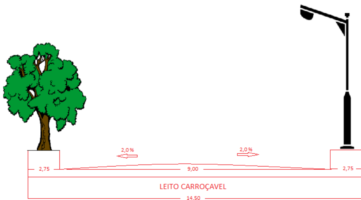
Figura 4. Corte Transversal das Ruas de 14,50 metros.
