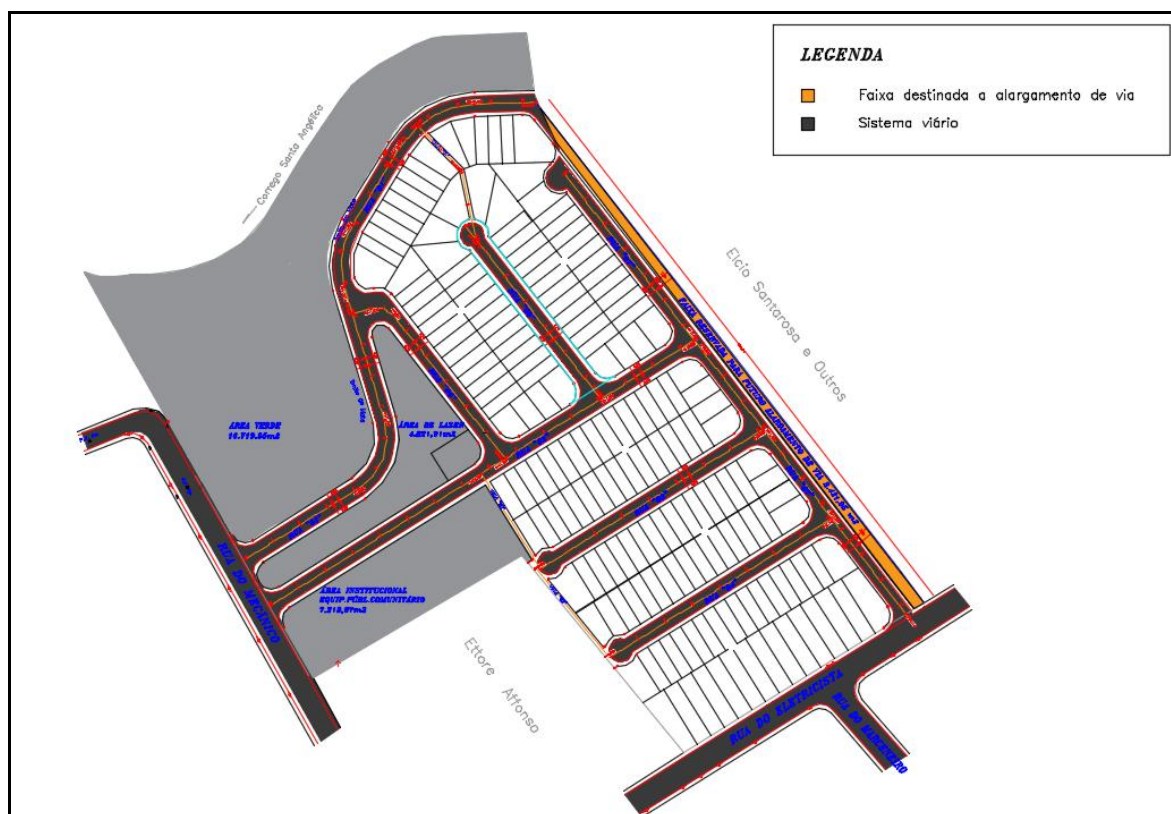
Figura 6. Configuração final do sistema viário (anexo ao relatório em folha A1)
